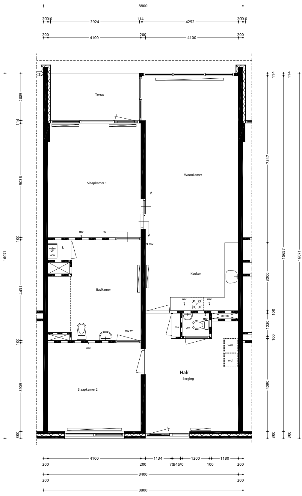
Plattegrond
